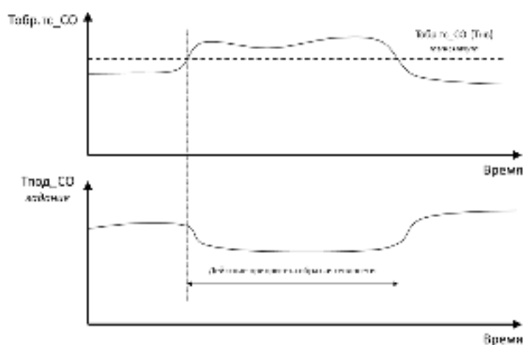
Рис. 44. Схема алгоритма ограничения T_{под\_СО} по обратной температуре теплосети.
