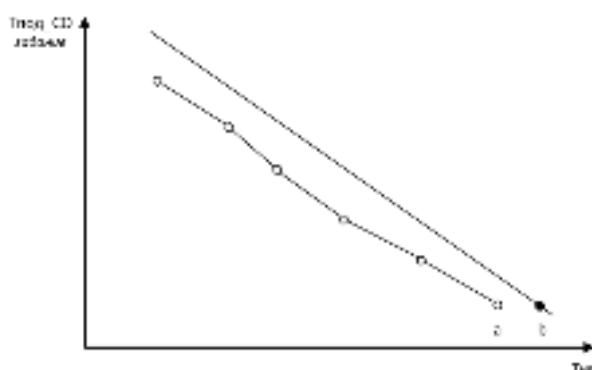
Рис.41. Два варианта задания отопительного графика: график по точкам (a) и через угол наклона (b).
